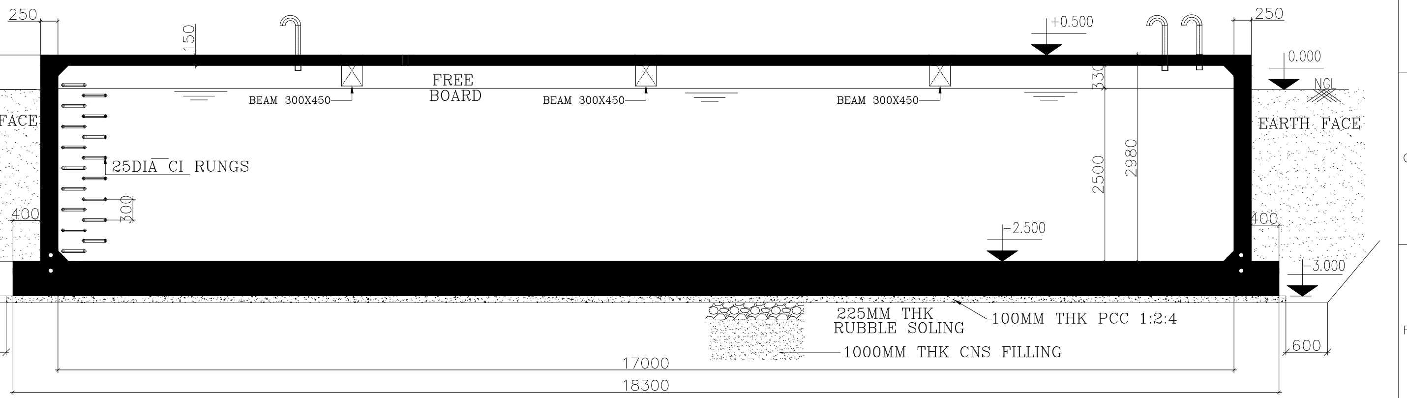
SECTION A-A
