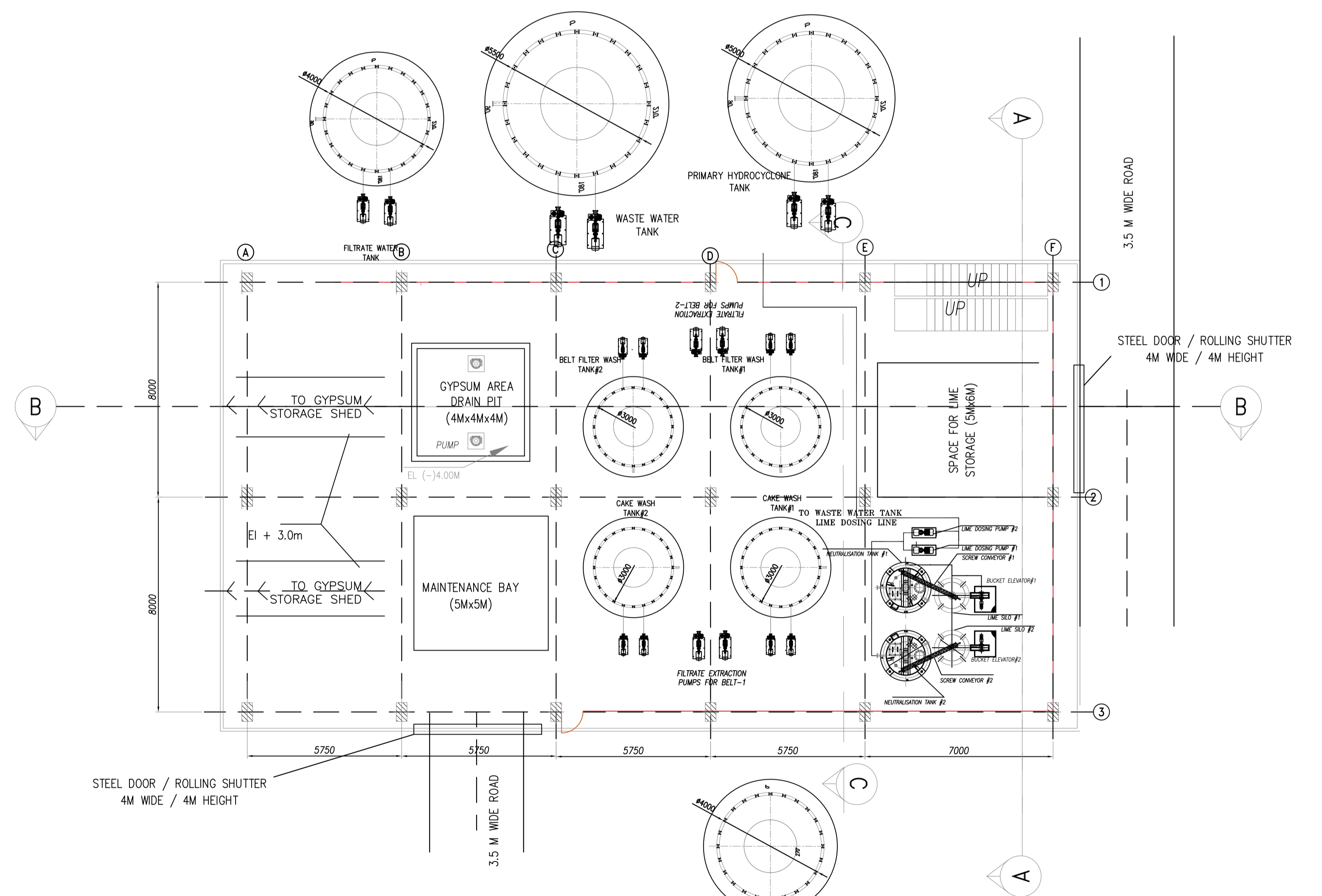
PLAN @ EL(±)0.00M
