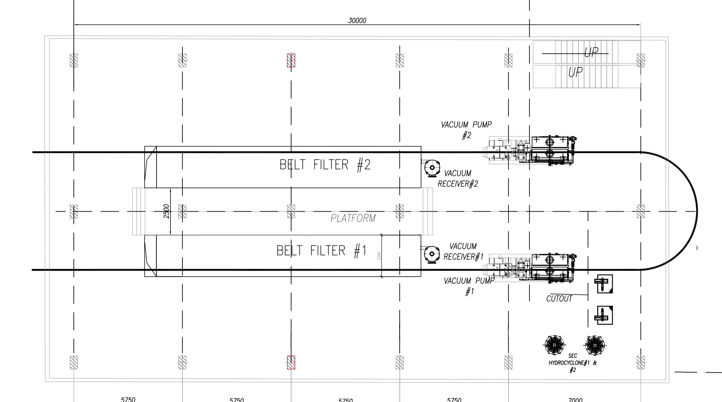
PLAN @ EL (+) 9.00M
